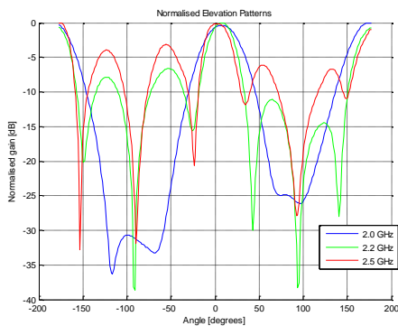
Elevation (E-Plane)
